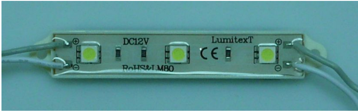
3-5050-SW57 LumiString LED module met 3 witte 5050 SMD LEDs met Epistar chips.
